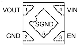
ZQFN-4L 1x1 (ZDFN-4L 1x1)
